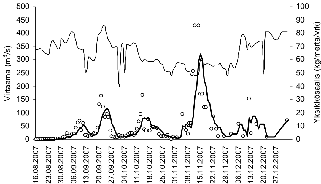
Kuva 5. Kymijoen vuorokausivirtaama (Mylykoski, ohut viiva) ja nahkiaispyynnin päiväkohtaiset keskimääräiset yksikkösaaliit (kg/m 3 /vrk., vaaleat täplät) vuonna 2007 sekä yksikkösaaliin liukuva keskiarvo (paksu viiva). Virtaamien ja nahkiaissaaliin välillä oli negatiivinen korrelaatio.
